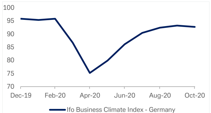
Grafico 1: Fiducia delle imprese tedesche misurata dall'indagine Ifo
