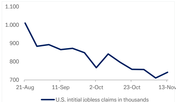
Grafico 2: Nuove richieste di sussidi di disoccupazione negli Stati Uniti
